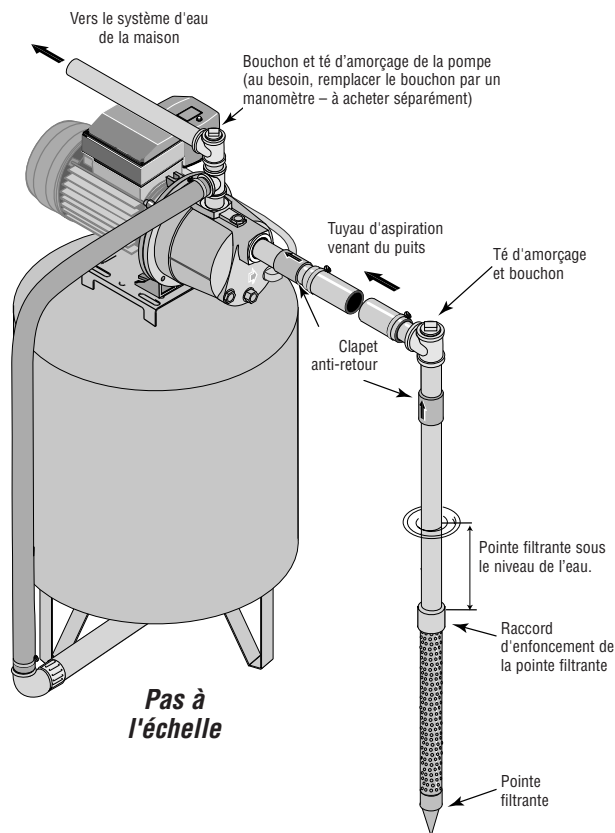
Figure 1: Installation avec une pointe filtrante
