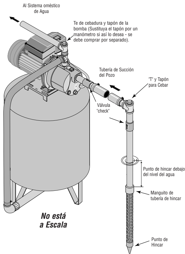
Figura 1 - Instalación del Punto de Hincar
