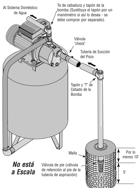
Figura 3: Instalación para agua superficial
