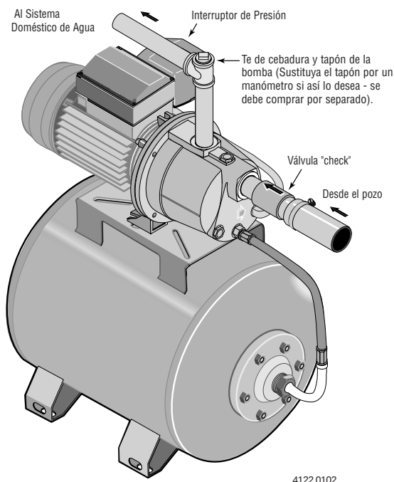
Figura 5 - Conexiones de la bomba sobre tanque.
